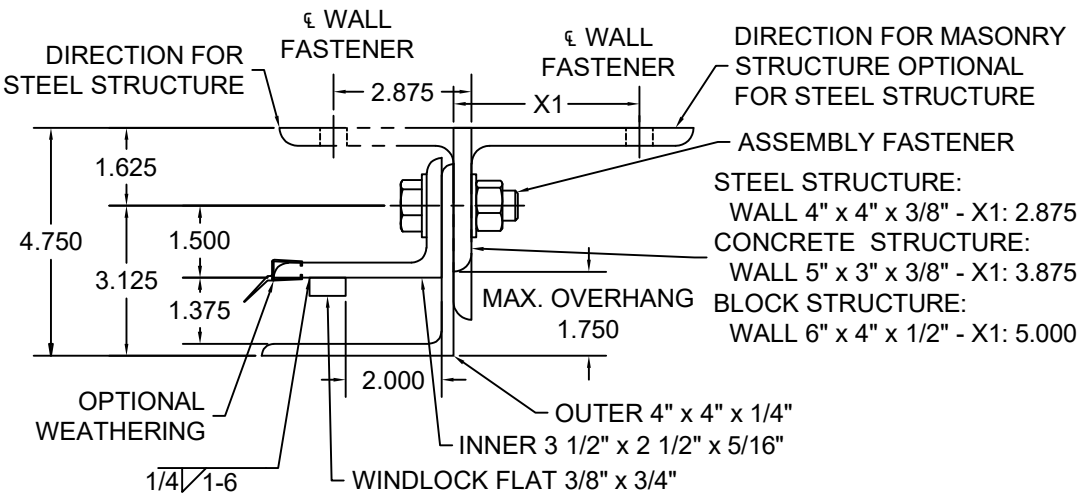
GUIDE ASSEMBLY TYPE DC 5 SCALE: 3" = 1'-0"
