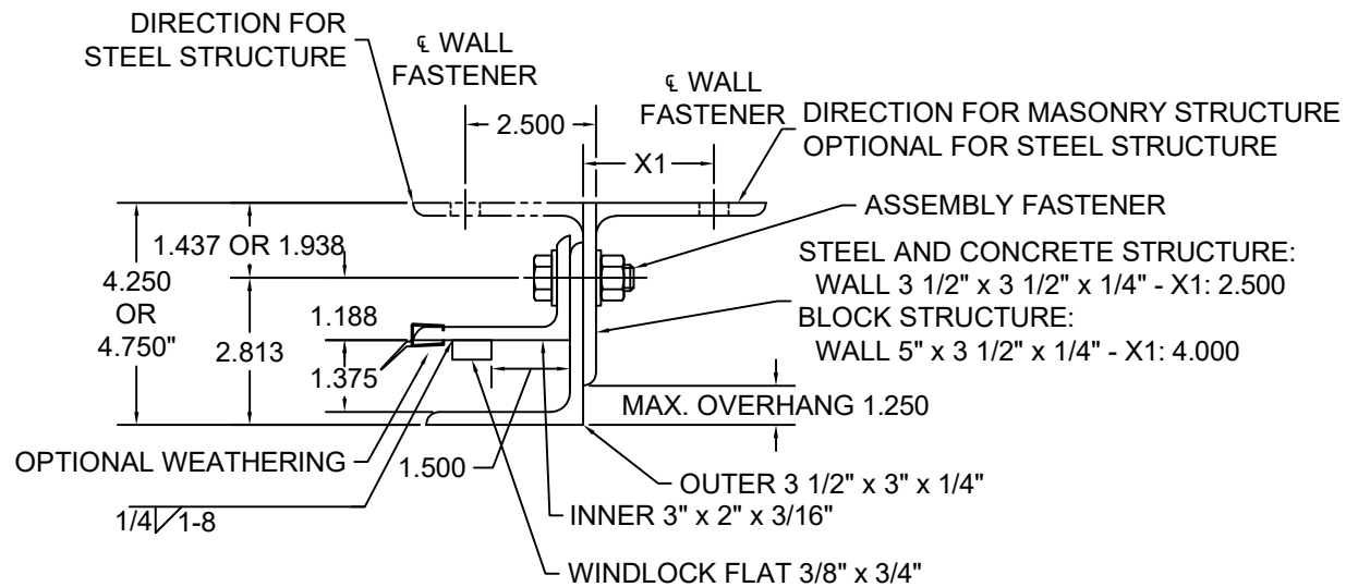
GUIDE ASSEMBLY TYPE DC 4 SCALE: 3" = 1'-0"
