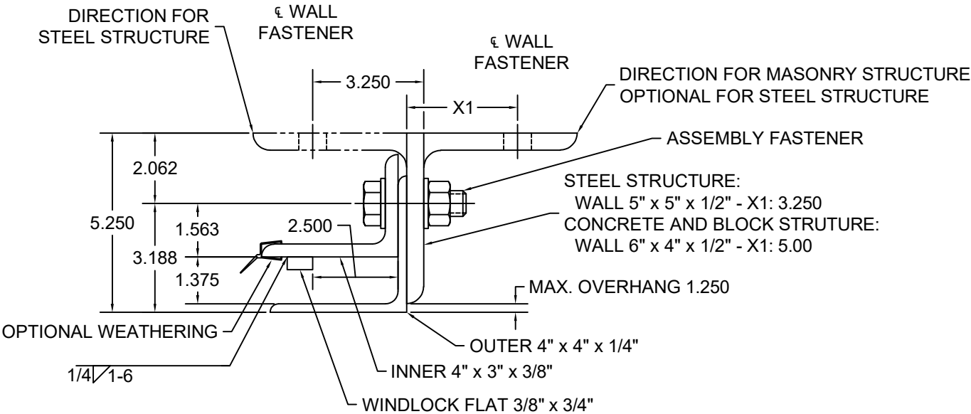
GUIDE ASSEMBLY TYPE DC 6 SCALE: 3" = 1'-0"
